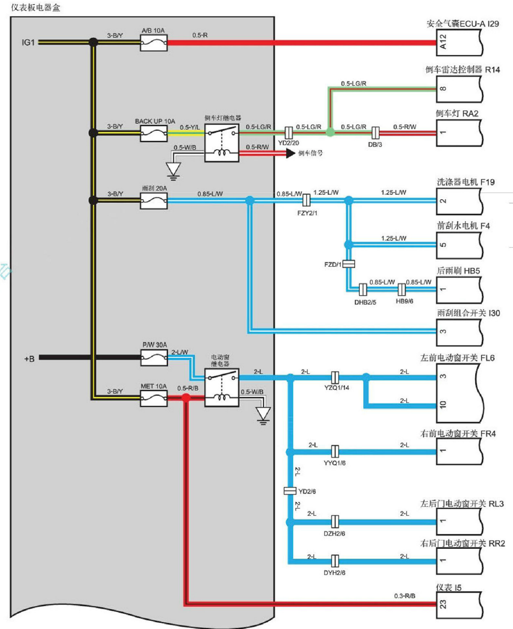
电源分配 (6/7)
